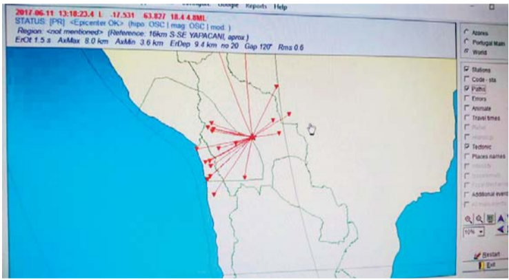
SISMO REGISTRADO POR EL OBSERVATORIO SAN CALIXTO.
